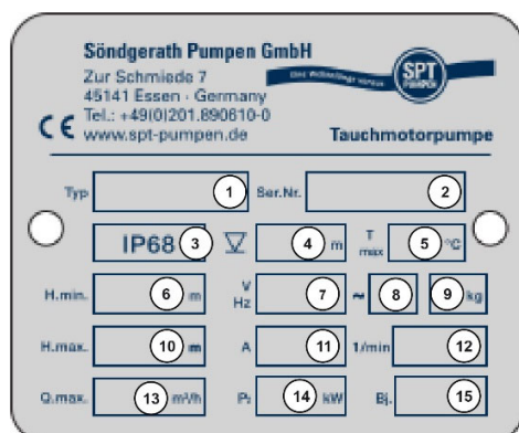
Abb. 1 Typenschild, Variante 1
