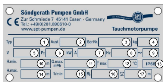
Abb. 3 Typenschild, Variante 3
