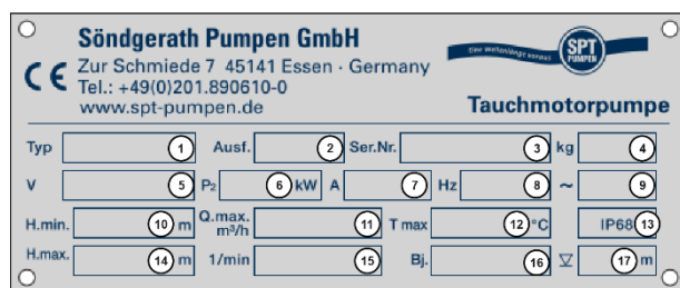
Obr. 4. Typový štítek, varianta 2
