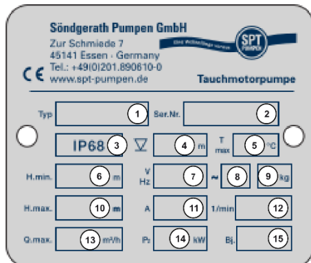
Afb. 1 Typeplaatje, variant 1
